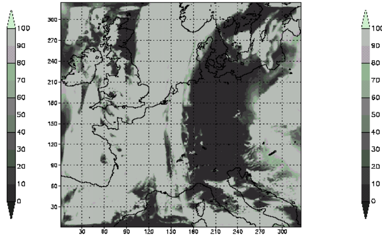
An. Moisture Incr. [kg/m^2], L 1, Feb 9, 2003
